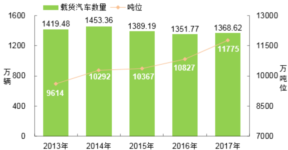
图 6 2013—2017 年全国载货汽车拥有量
