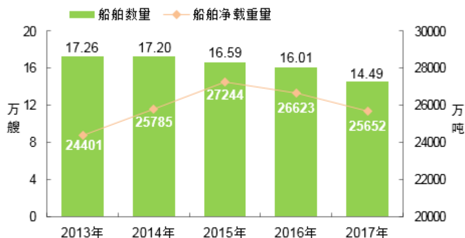
图 7 2013—2017 年全国水上运输船舶拥有量
