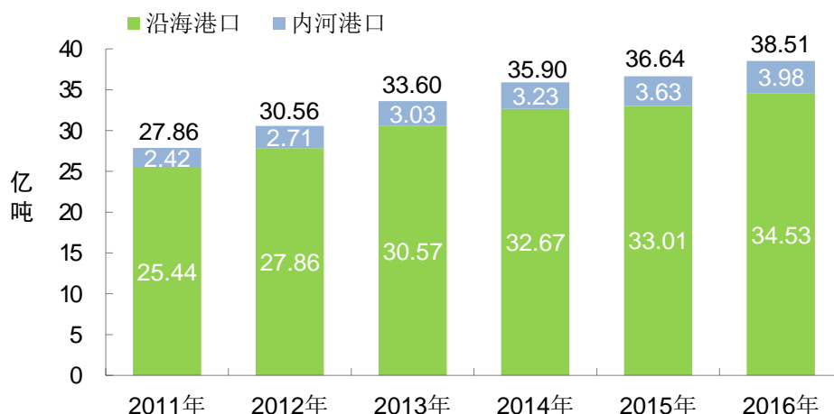
图 13 2011—2016 年全国港口外贸货物吞吐量
